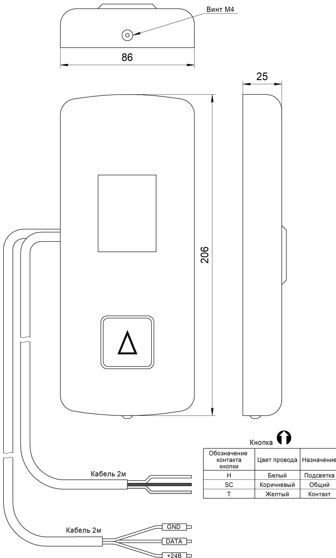
Рис.1 Внешний вид и габаритные размеры Вызывного поста ВВ-1001-1074-27
